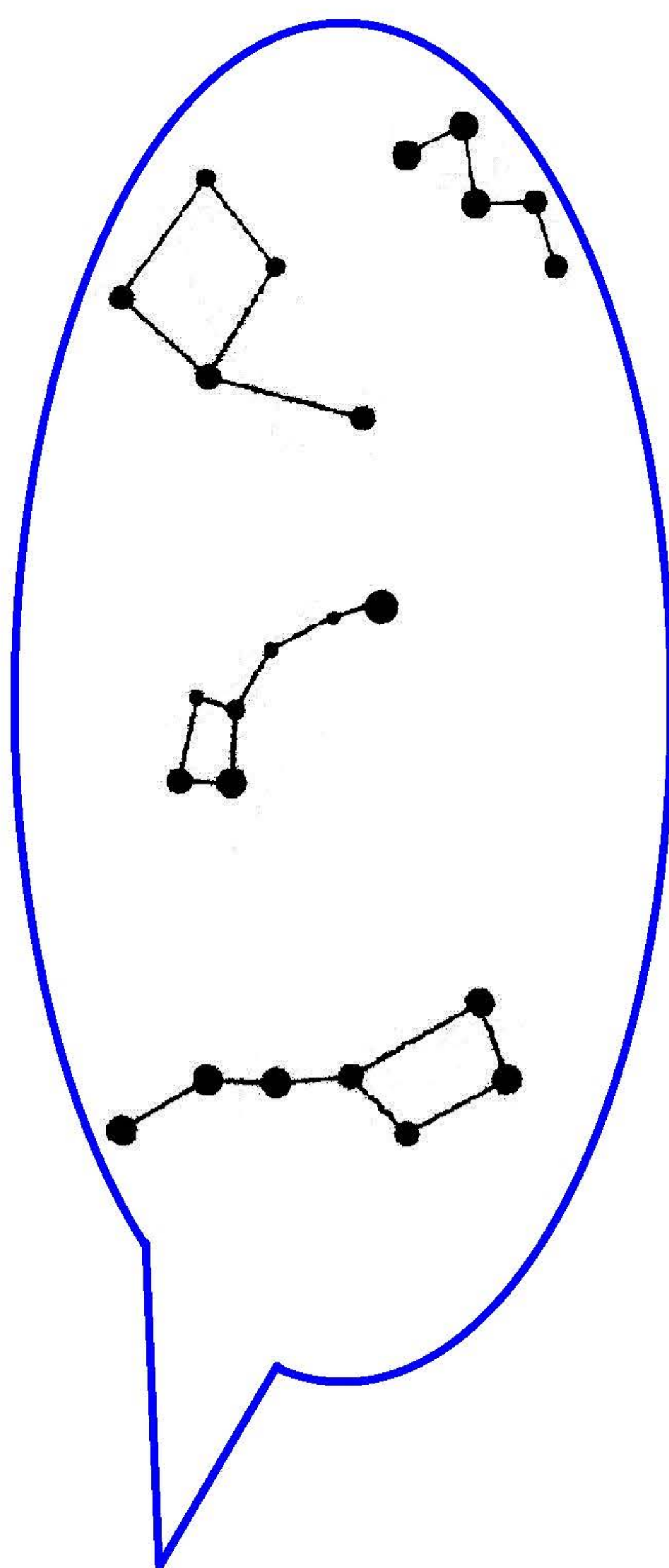
Zirkumpolarsternbilder
