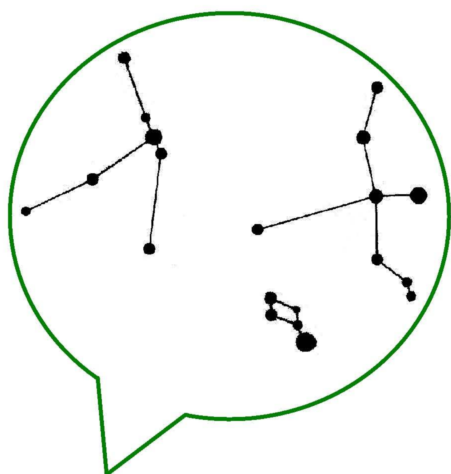
Sommer-Sternbilder
